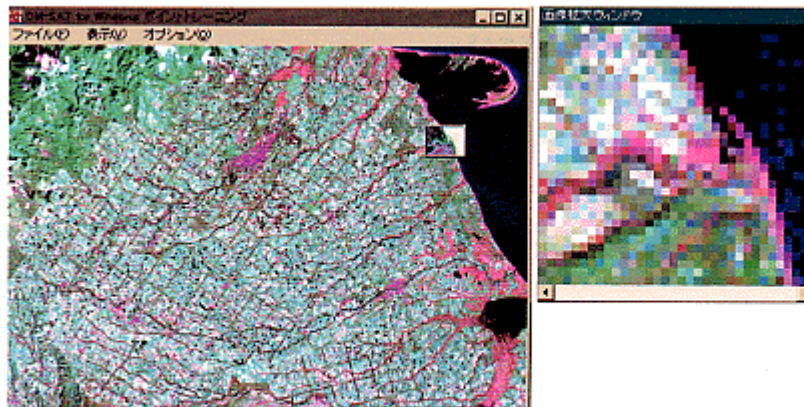
図6 北海道網走地方のMSS画像(58×46kmの範囲) 1981年11月5日の解像率2のMSS画像。画像の右上が町付野、右下が気連湖にあたる。中央部の格子状の道路である。リモートセンシング画像はタイル状のようなもので、画像を拡大していくと最後には四角形の集合になる。右側のウィンドウは、衛星観測値を拡大したもので、一つの四角形をピクセル(画素)という。
