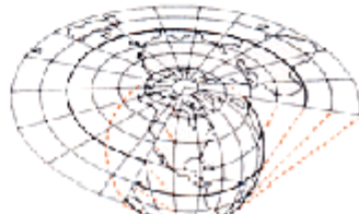
a) ランベルト正積方位図法
