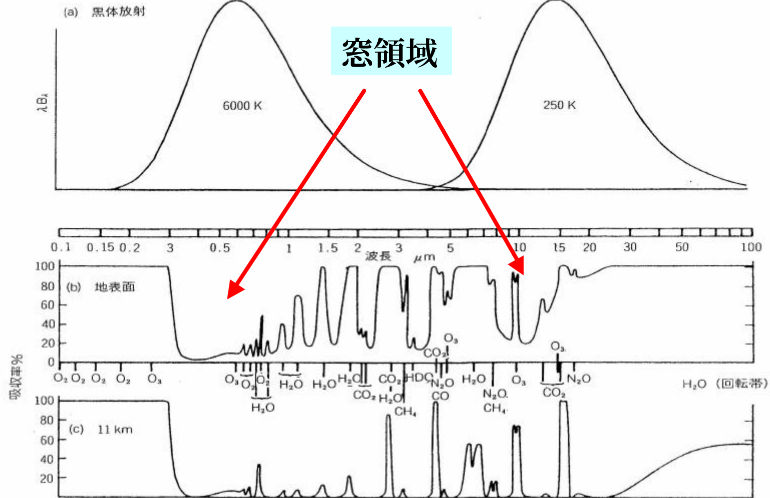
図 2.1.5 6000K と 250K の黒体放射スペクトル(a)と気体の吸収帯構造(b) (Goody and Yung, 1989).
